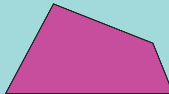
quadrilateral
